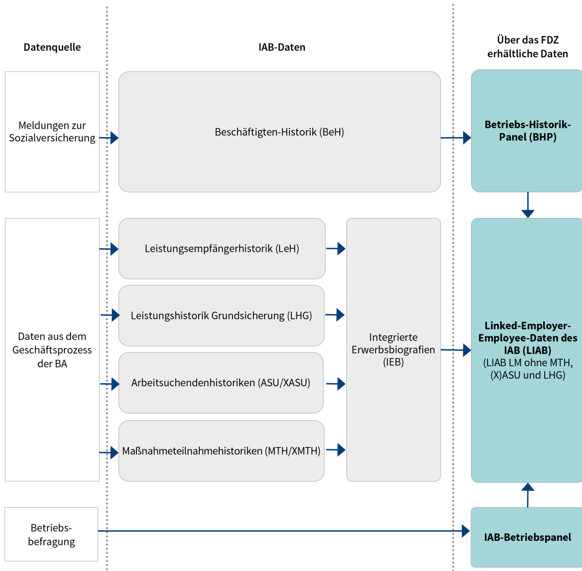
Abbildung 3: Quellen des LIAB
