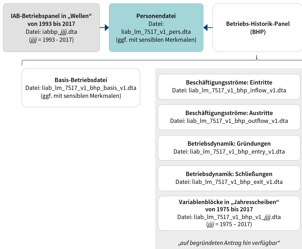
Abbildung 2: Datenhaltung der Linked-Employer-Employee-Daten im LIAB LM 7517
